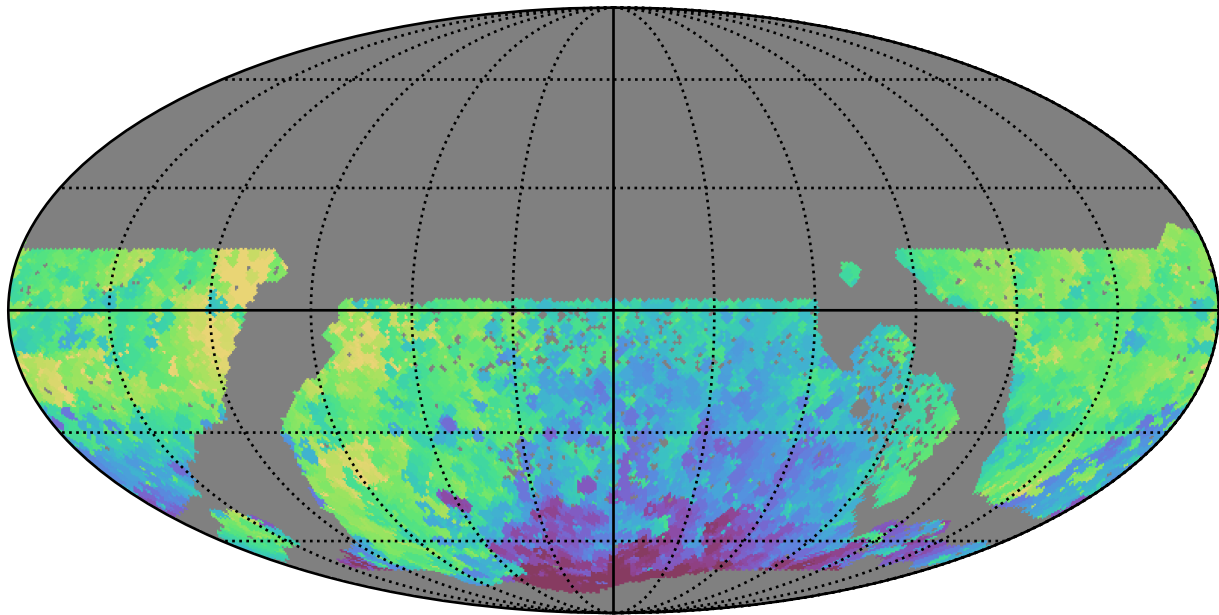
baseline_v3.3_10yrs WFD y band: Min HA
