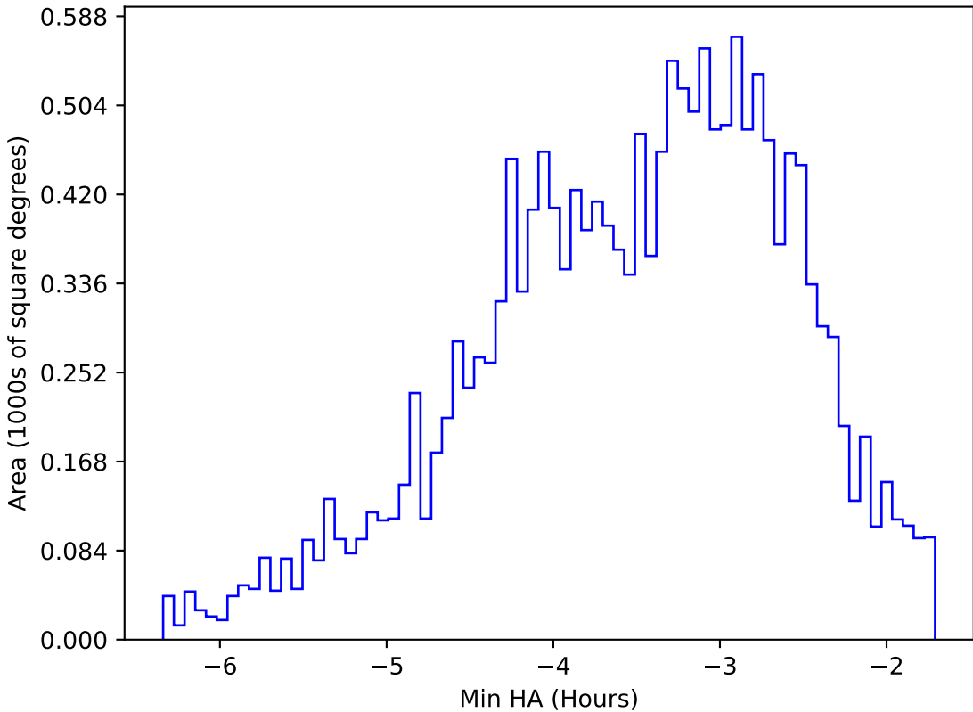
baseline_v3.3_10yrs WFD y band: Min HA
