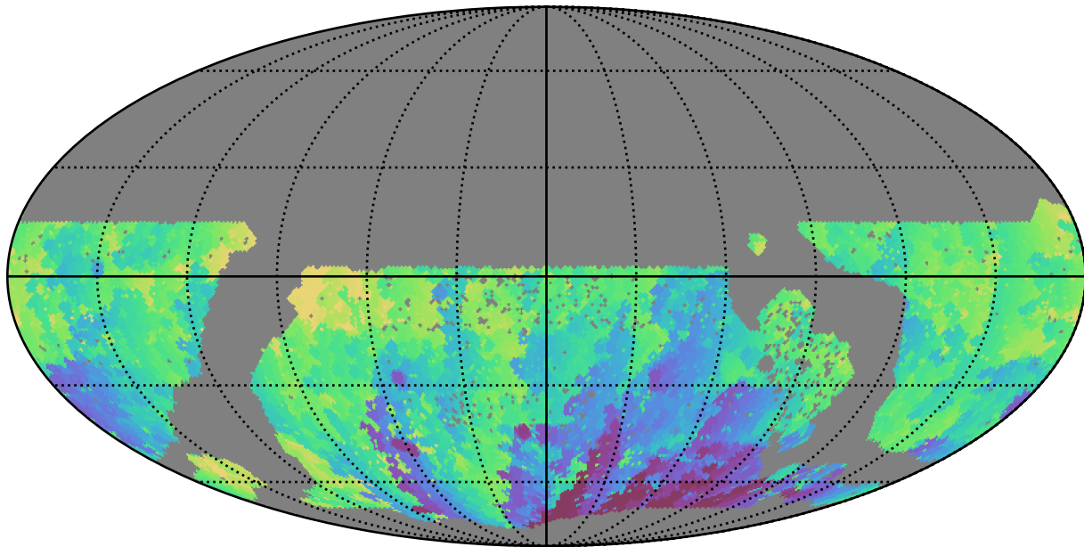
baseline_v3.3_10yrs WFD u band: Min HA
