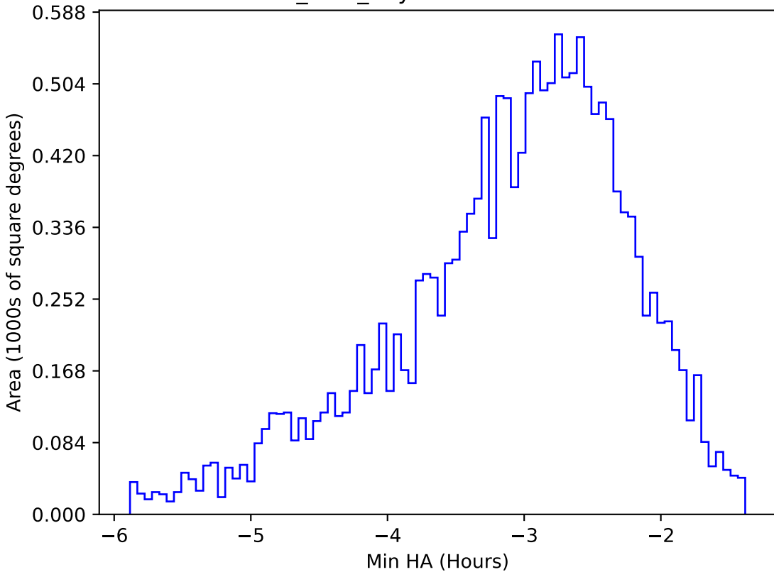
baseline_v3.3_10yrs WFD u band: Min HA
