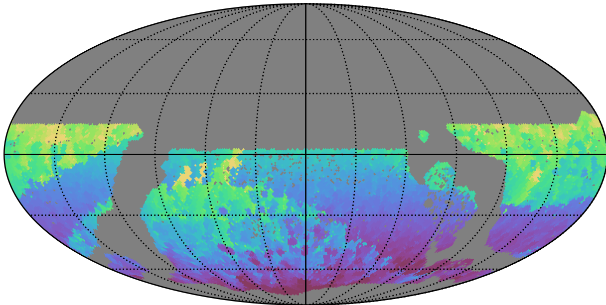
baseline_v3.3_10yrs WFD r band: Min HA
