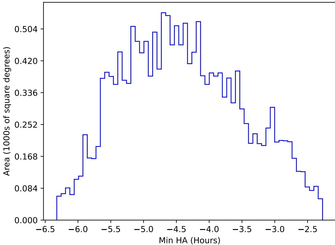
baseline_v3.3_10yrs WFD r band: Min HA
