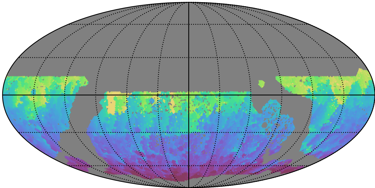
baseline_v3.3_10yrs WFD g band: Min HA
