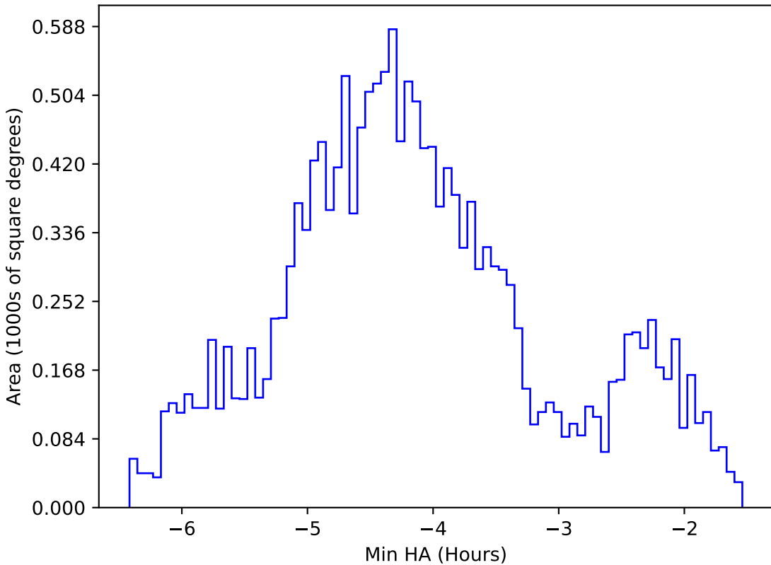
baseline_v3.3_10yrs WFD g band: Min HA
