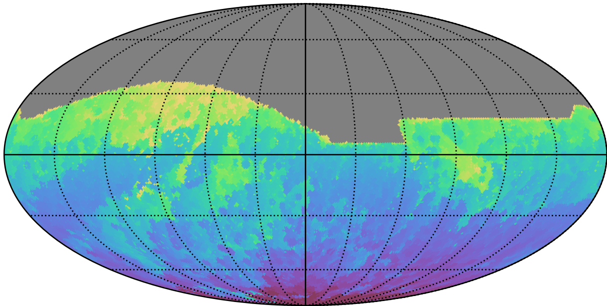
baseline_v3.3_10yrs All sky z band: Min HA
