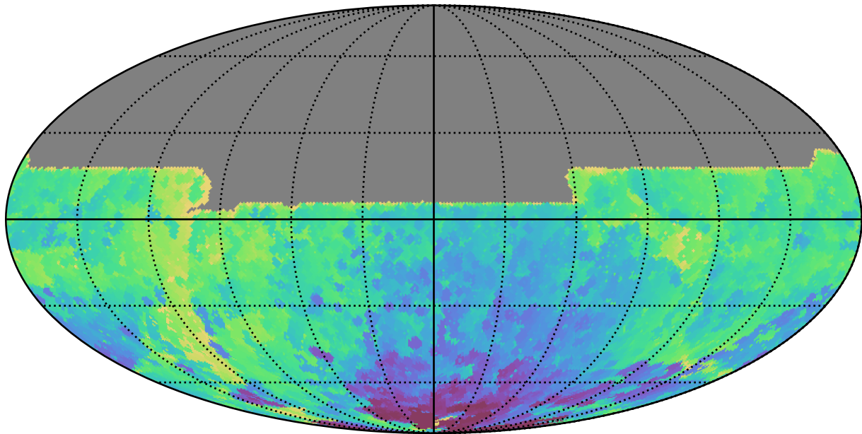
baseline_v3.3_10yrs All sky y band: Min HA
