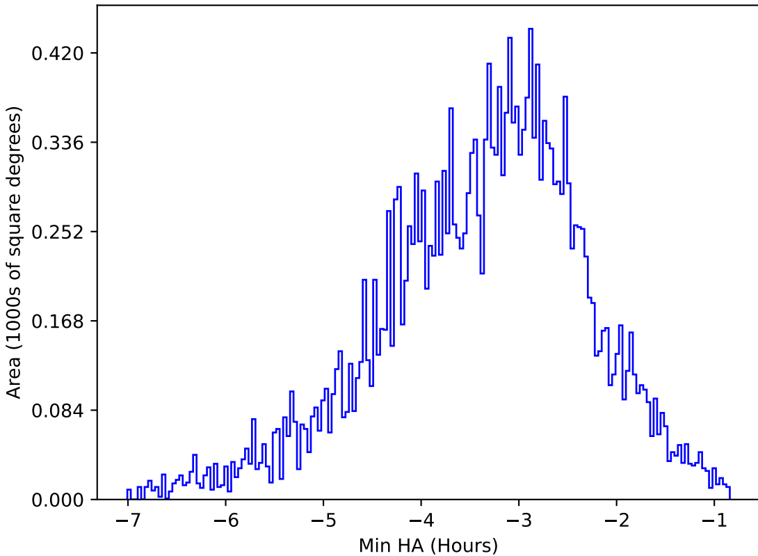
baseline_v3.3_10yrs All sky y band: Min HA
