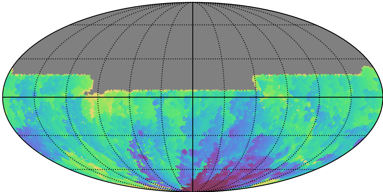
baseline_v3.3_10yrs All sky u band: Min HA
