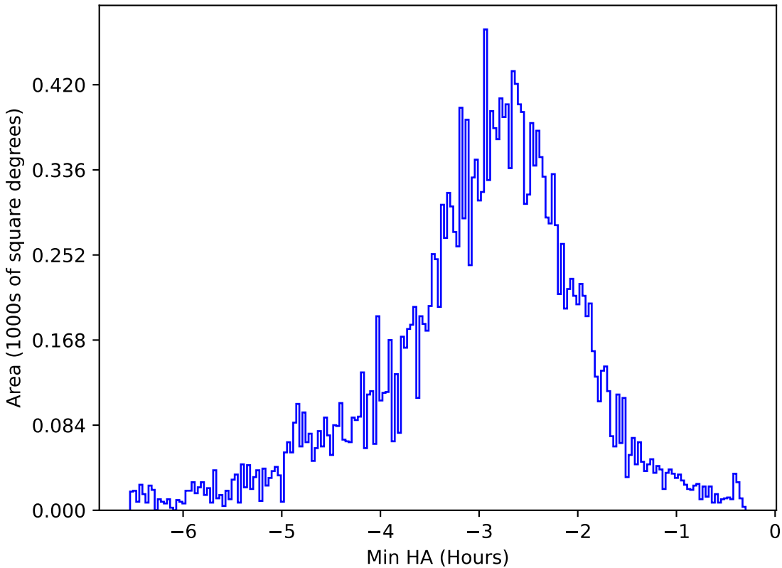
baseline_v3.3_10yrs All sky u band: Min HA
