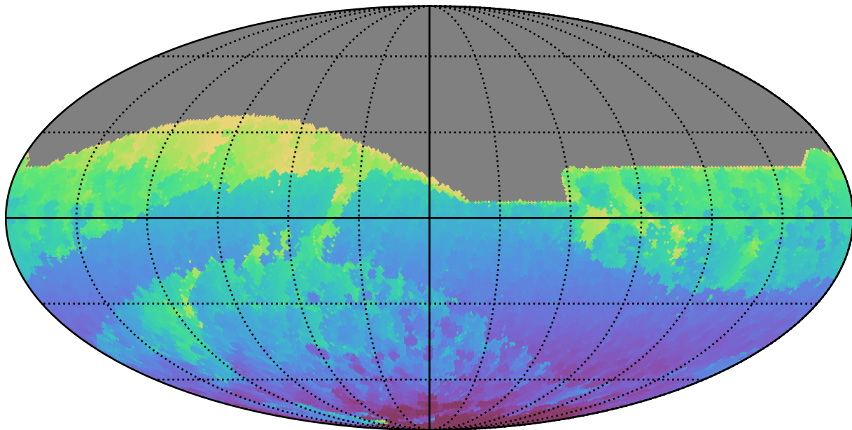
baseline_v3.3_10yrs All sky r band: Min HA
