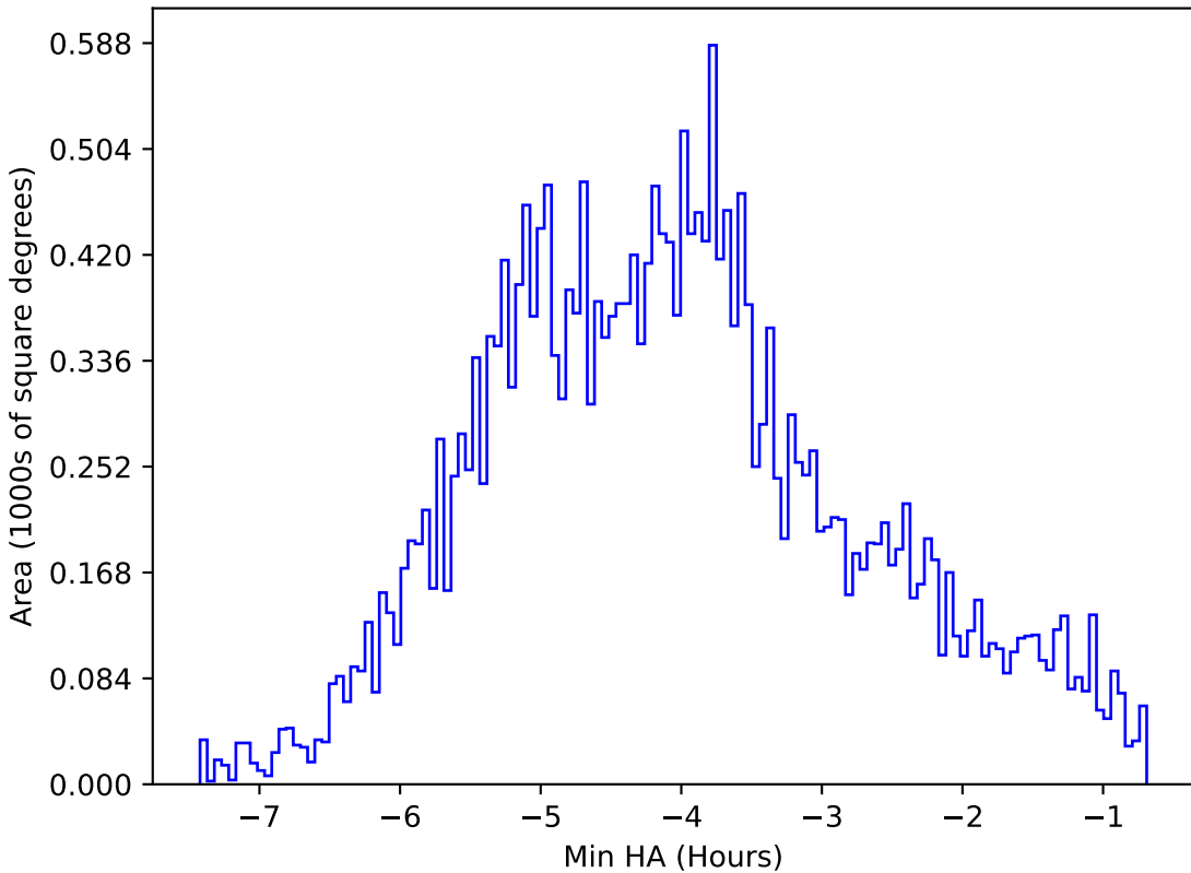
baseline_v3.3_10yrs All sky i band: Min HA
