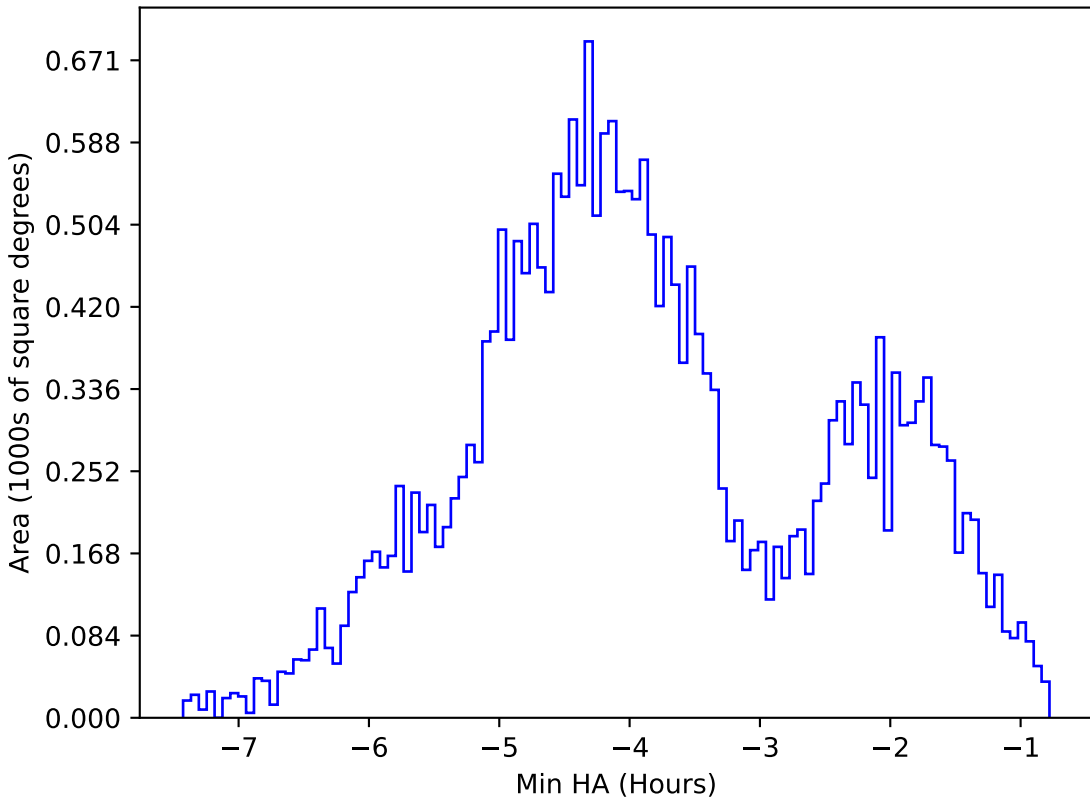
baseline_v3.3_10yrs All sky g band: Min HA
