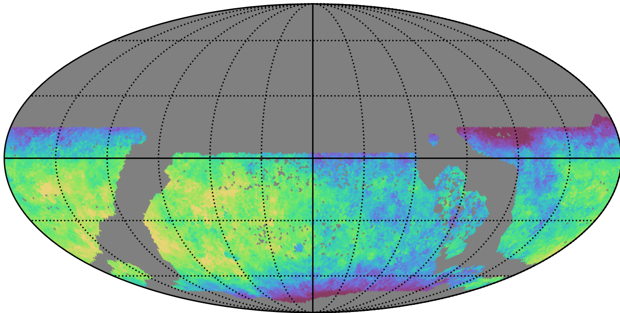
baseline_v3.3_10yrs WFD y band: Median saturation_mag
