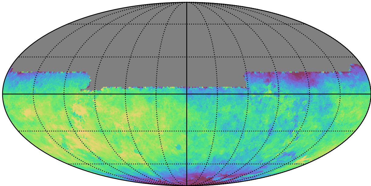
baseline_v3.3_10yrs All sky y band: Median saturation_mag
