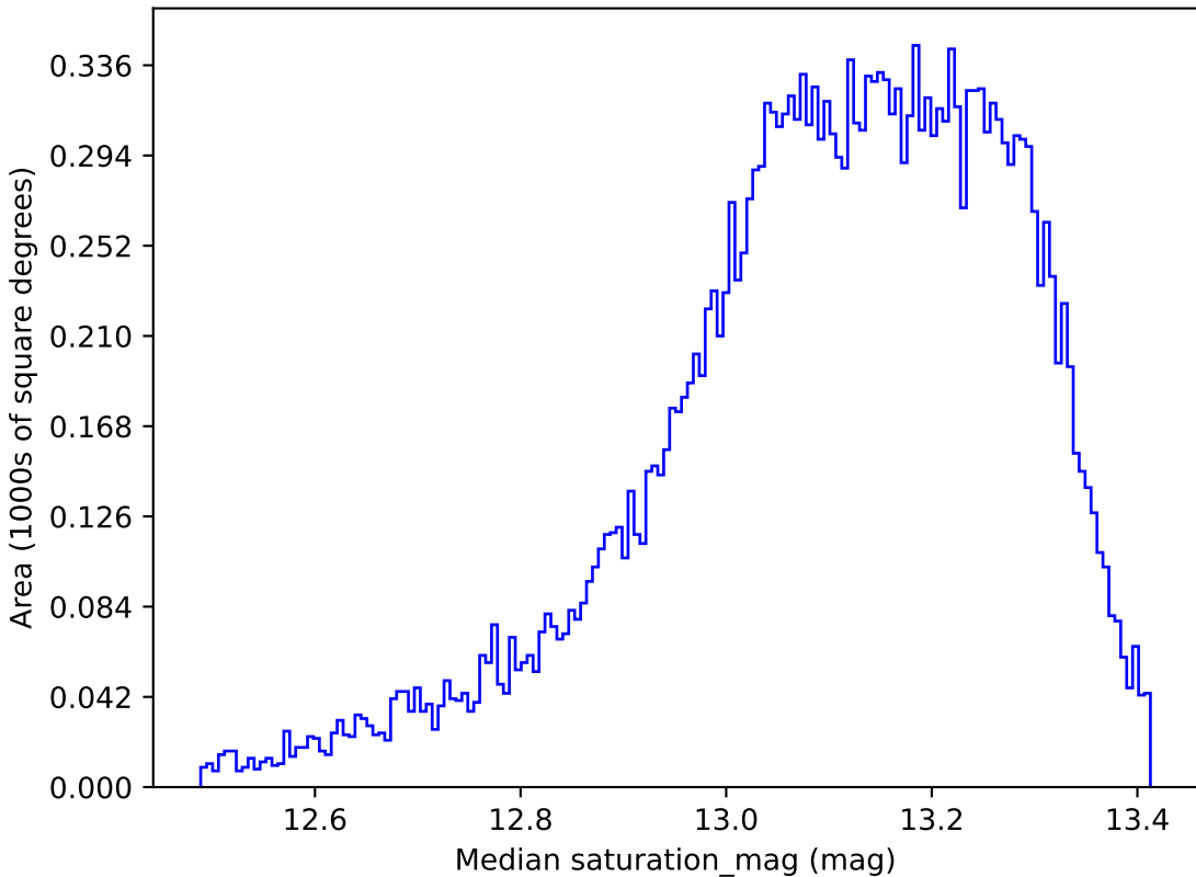
baseline_v3.3_10yrs All sky y band: Median saturation_mag
