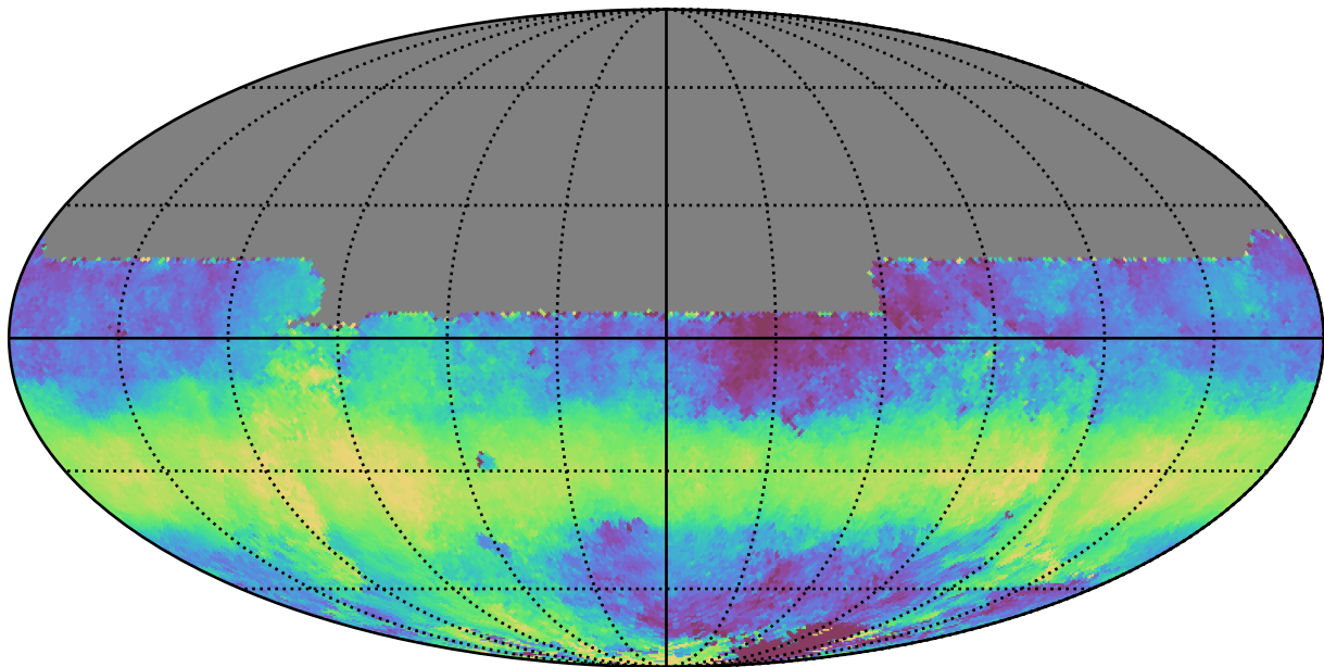
baseline_v3.3_10yrs All sky y band: Median HA
