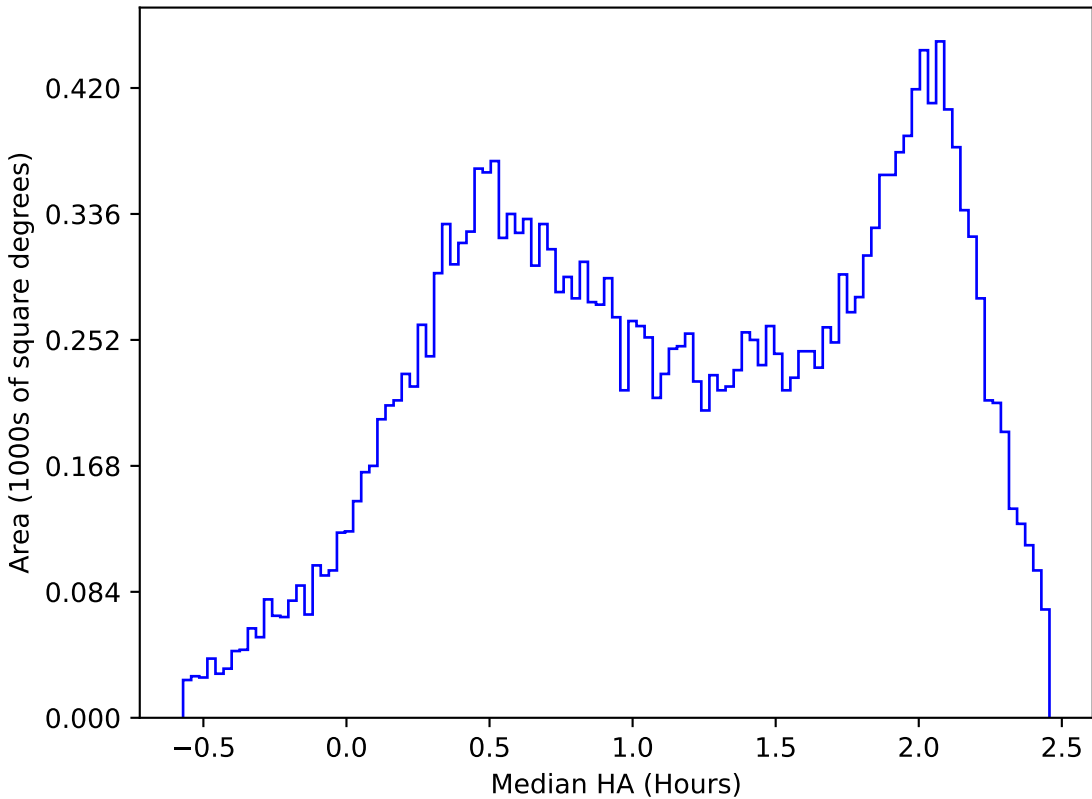
baseline_v3.3_10yrs All sky y band: Median HA
