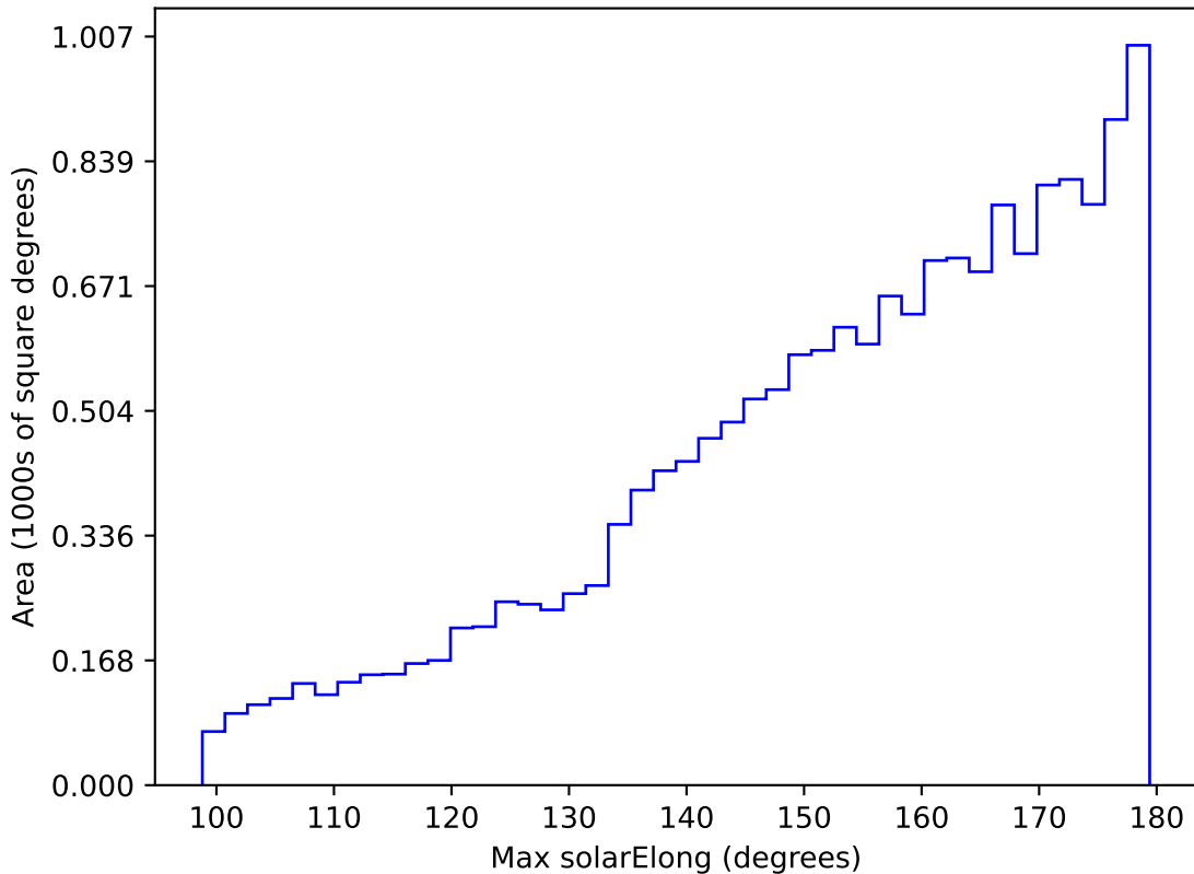
baseline_v3.3_10yrs WFD z band: Max solarElong
