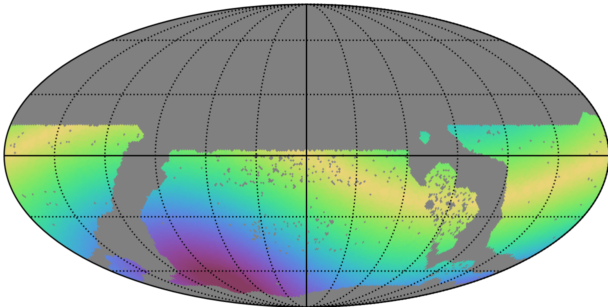
baseline_v3.3_10yrs WFD y band: Max solarElong
