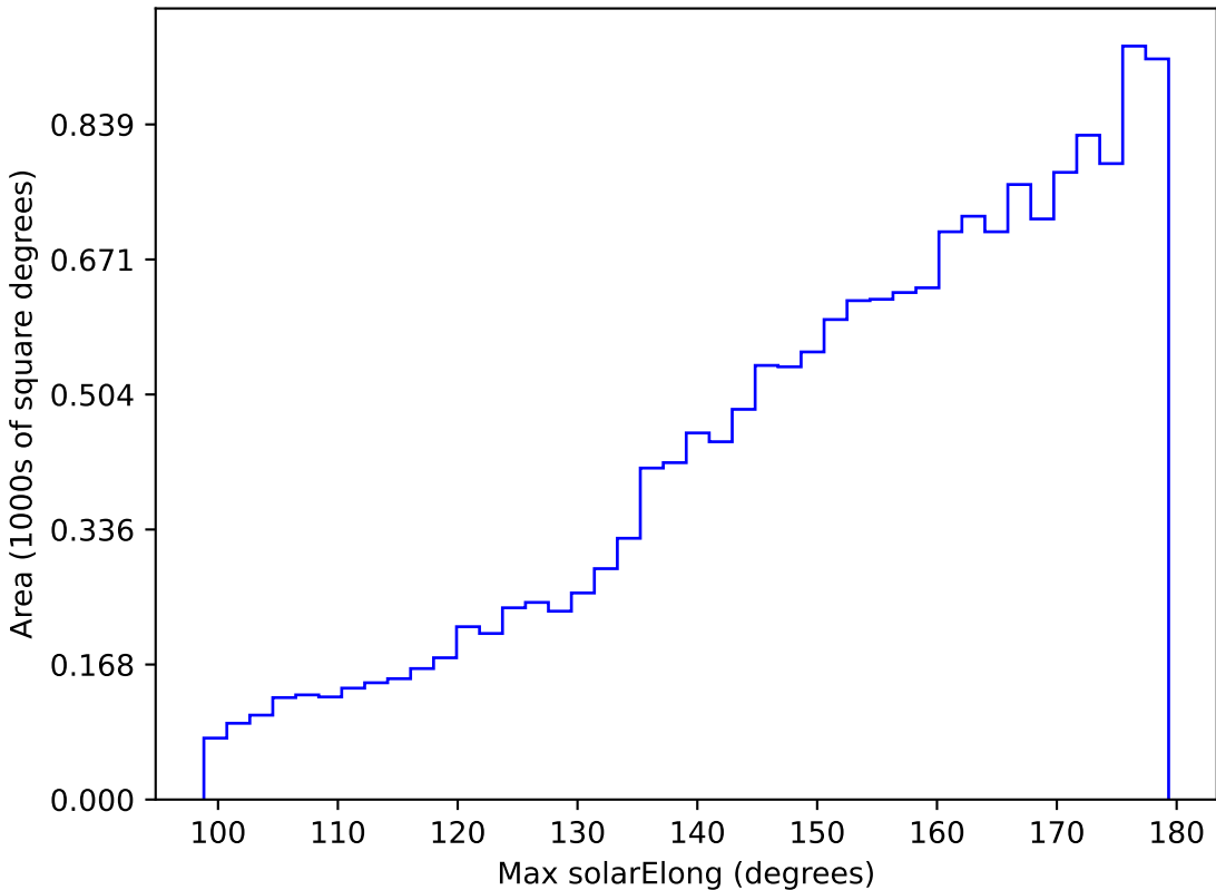
baseline_v3.3_10yrs WFD y band: Max solarElong
