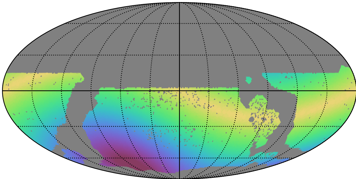
baseline_v3.3_10yrs WFD i band: Max solarElong
