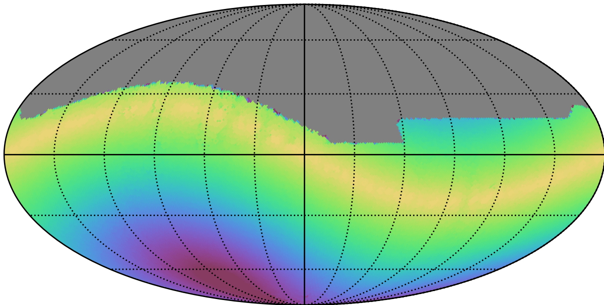
baseline_v3.3_10yrs All sky z band: Max solarElong
