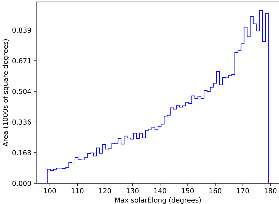
baseline_v3.3_10yrs All sky z band: Max solarElong
