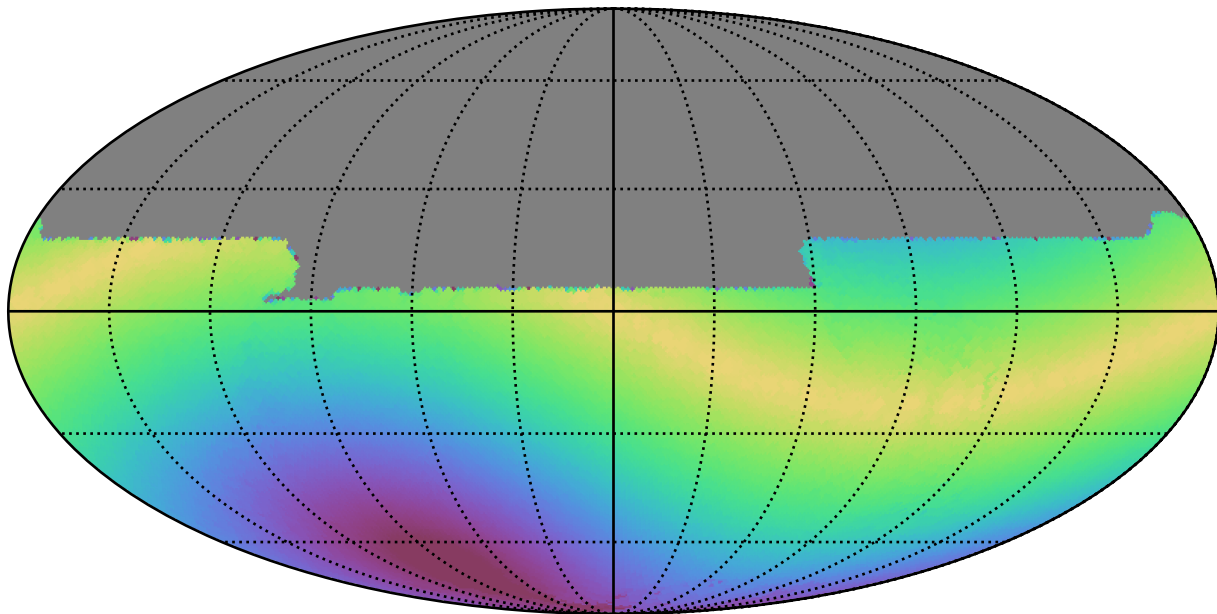
baseline_v3.3_10yrs All sky y band: Max solarElong
