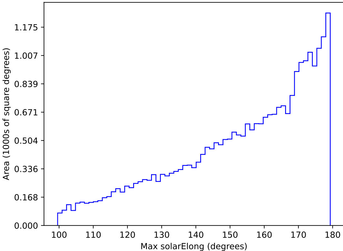
baseline_v3.3_10yrs All sky r band: Max solarElong
