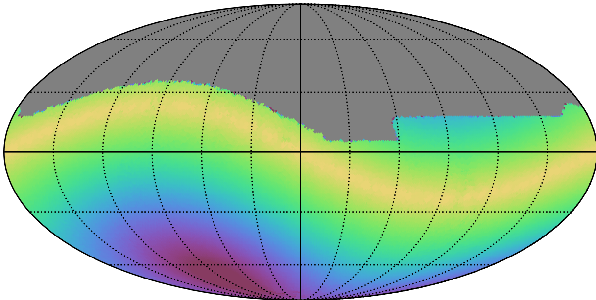
baseline_v3.3_10yrs All sky i band: Max solarElong
