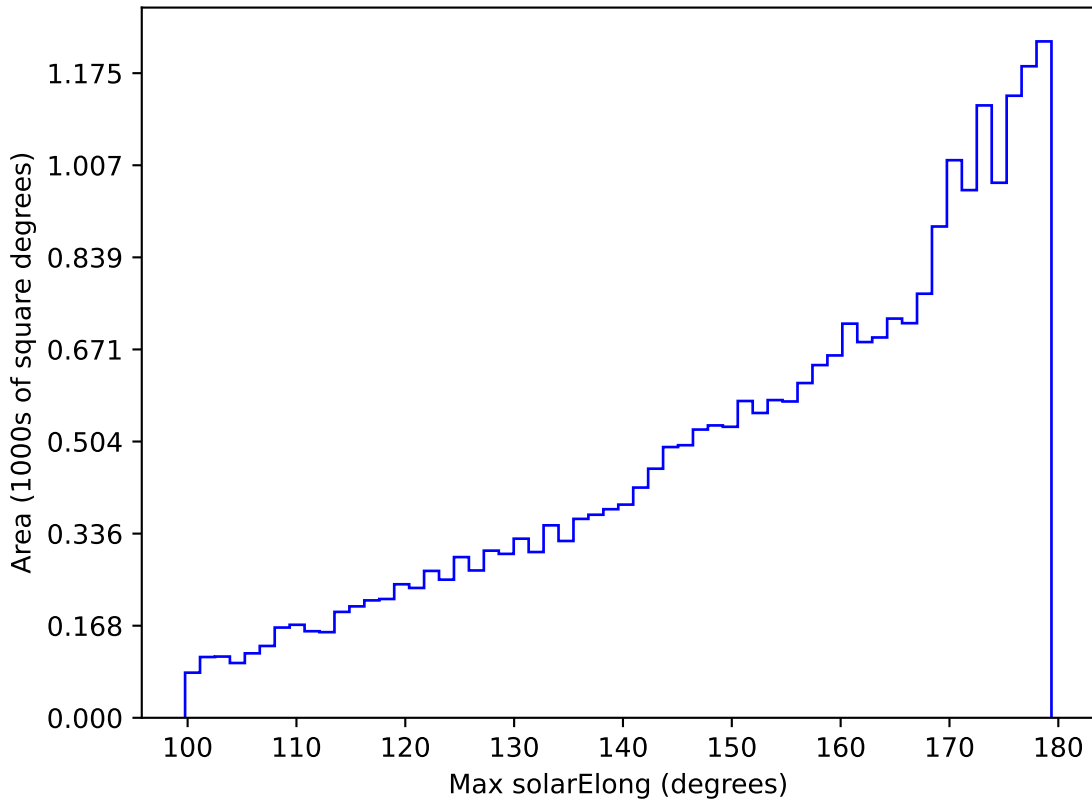
baseline_v3.3_10yrs All sky i band: Max solarElong
