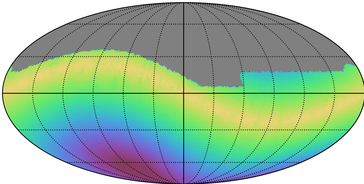
baseline_v3.3_10yrs All sky g band: Max solarElong
