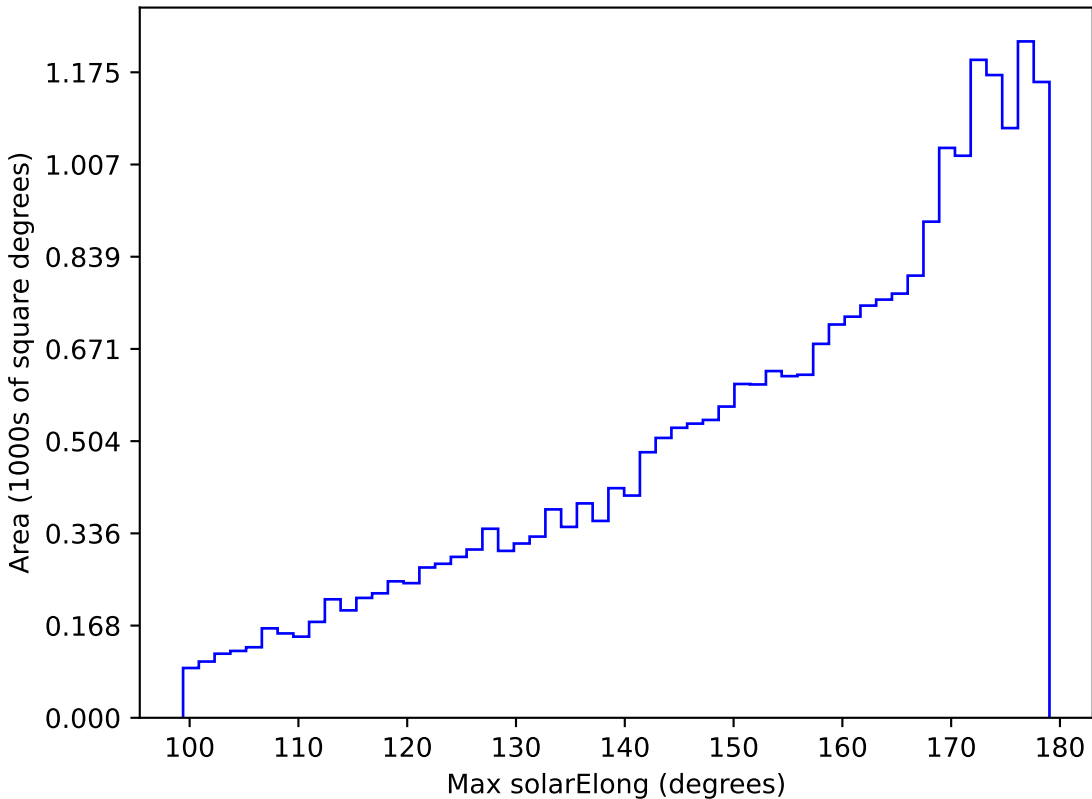
baseline_v3.3_10yrs All sky g band: Max solarElong
