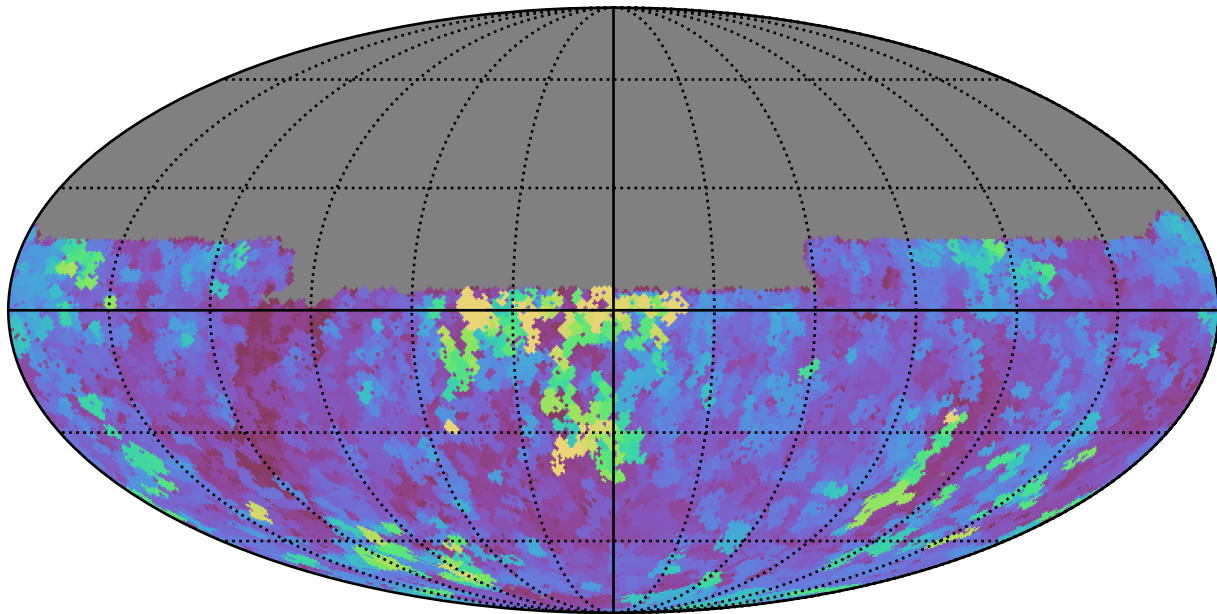
baseline_v3.3_10yrs Yr 1 y band: Max seeingGeom
