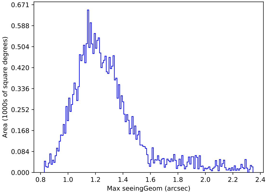
baseline_v3.3_10yrs Yr 1 y band: Max seeingGeom
