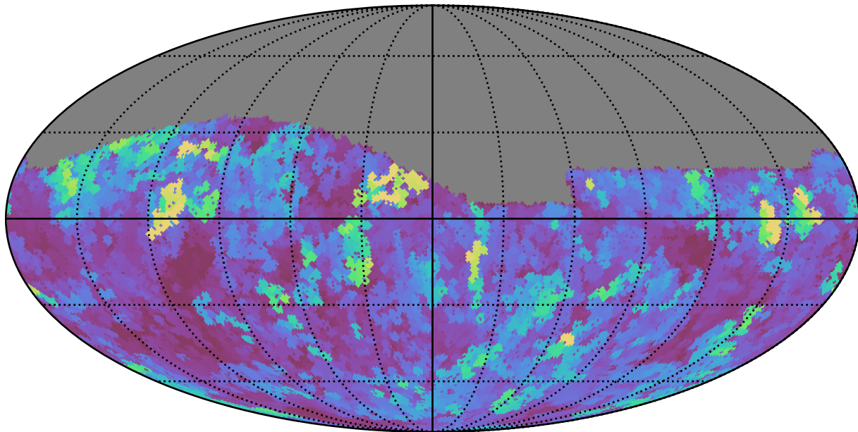
baseline_v3.3_10yrs Yr 1 i band: Max seeingGeom
