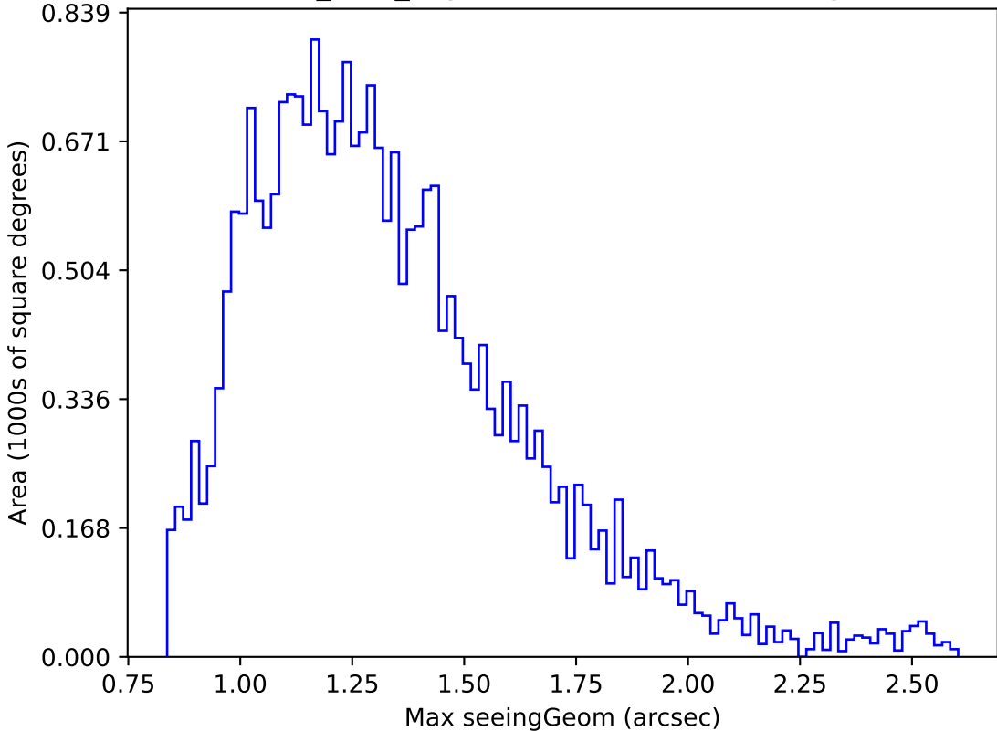
baseline_v3.3_10yrs Yr 1 i band: Max seeingGeom
