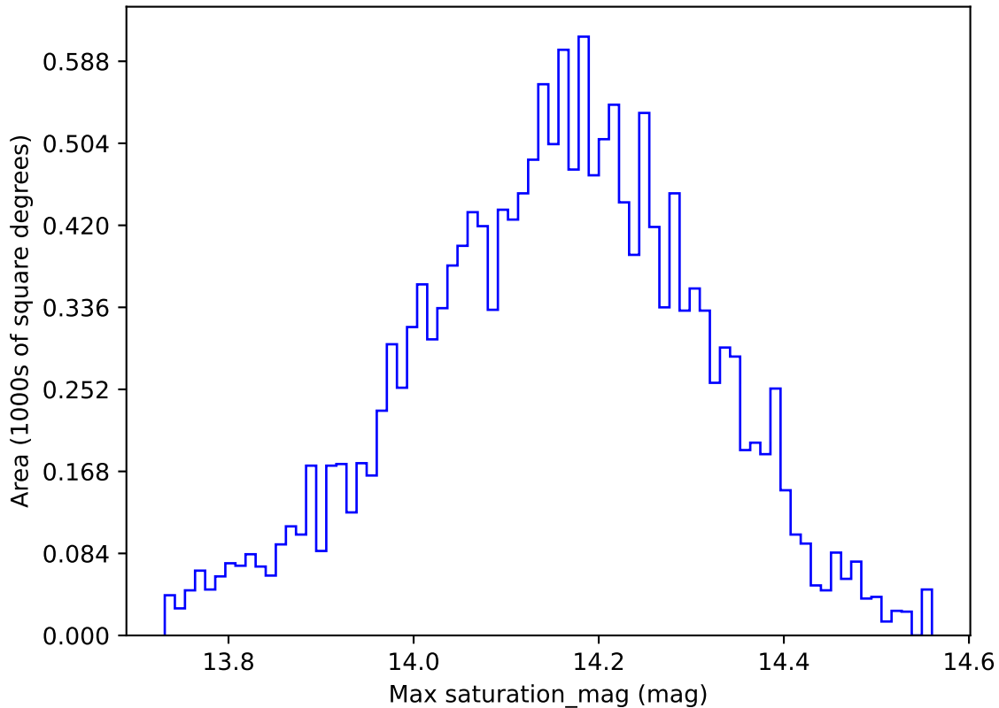
baseline_v3.3_10yrs WFD y band: Max saturation_mag
