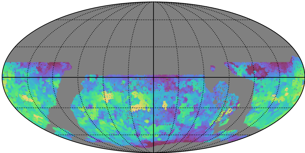
baseline_v3.3_10yrs WFD u band: Max saturation_mag
