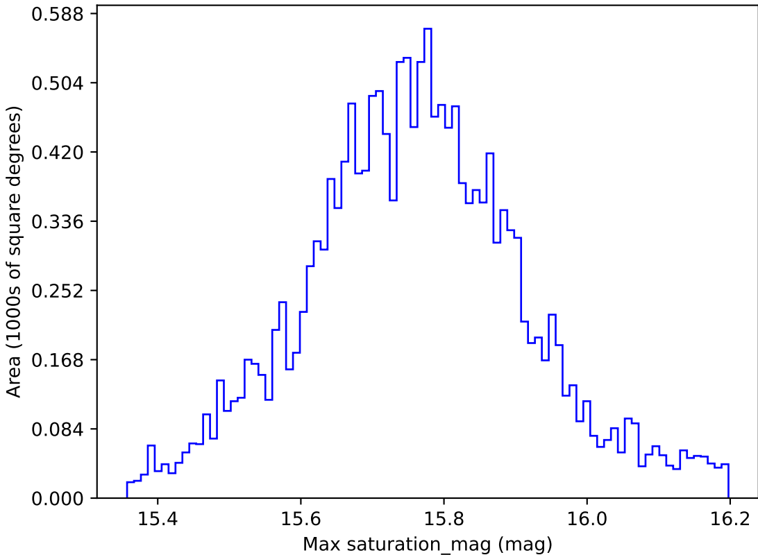
baseline_v3.3_10yrs WFD r band: Max saturation_mag
