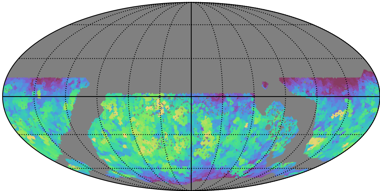
baseline_v3.3_10yrs WFD i band: Max saturation_mag
