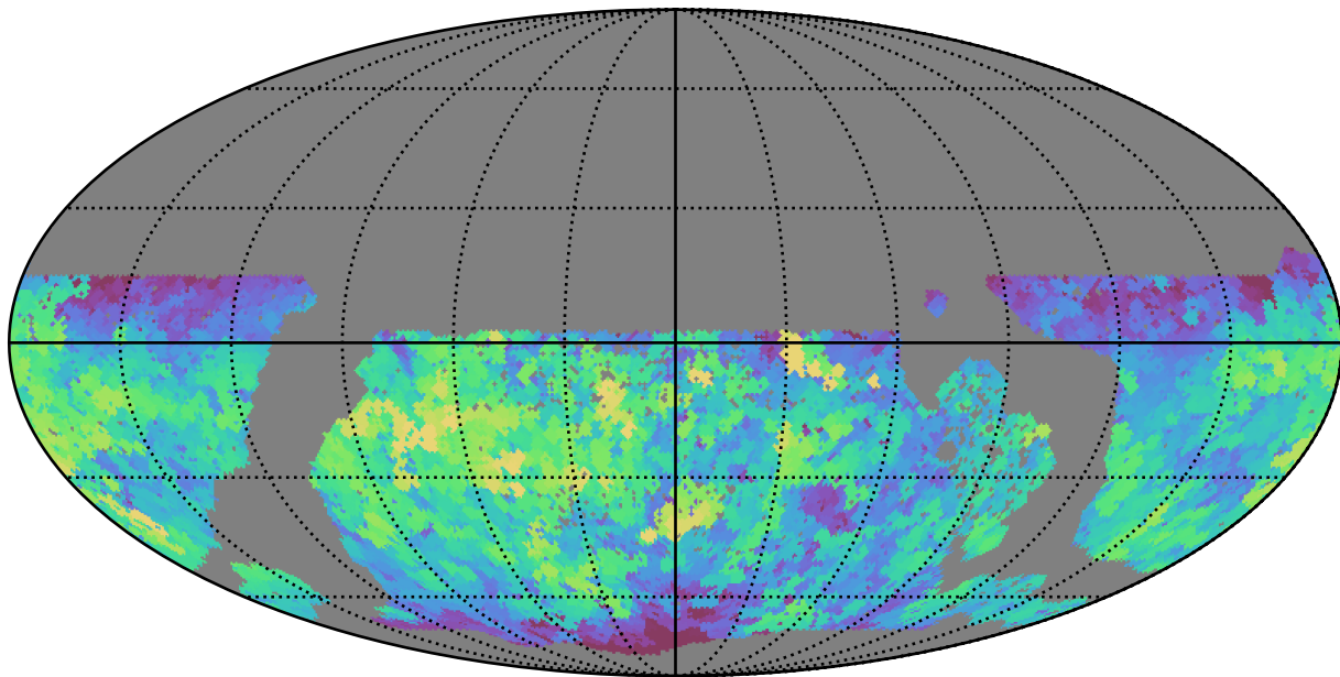
baseline_v3.3_10yrs WFD g band: Max saturation_mag
