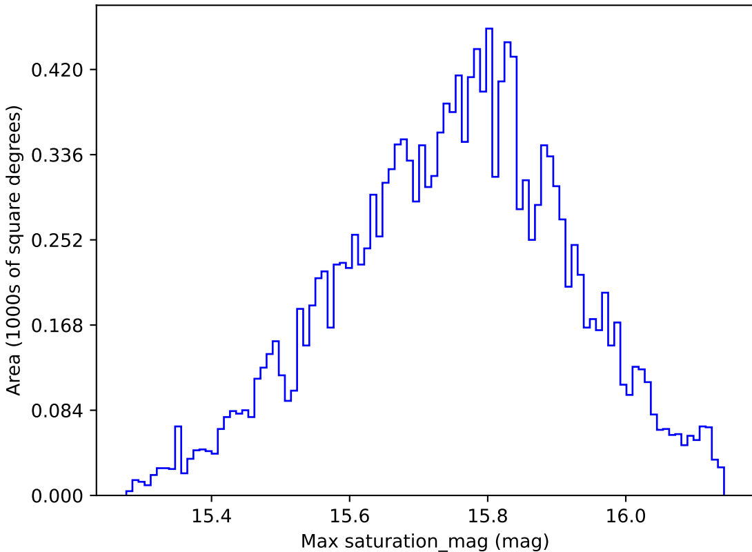
baseline_v3.3_10yrs WFD g band: Max saturation_mag
