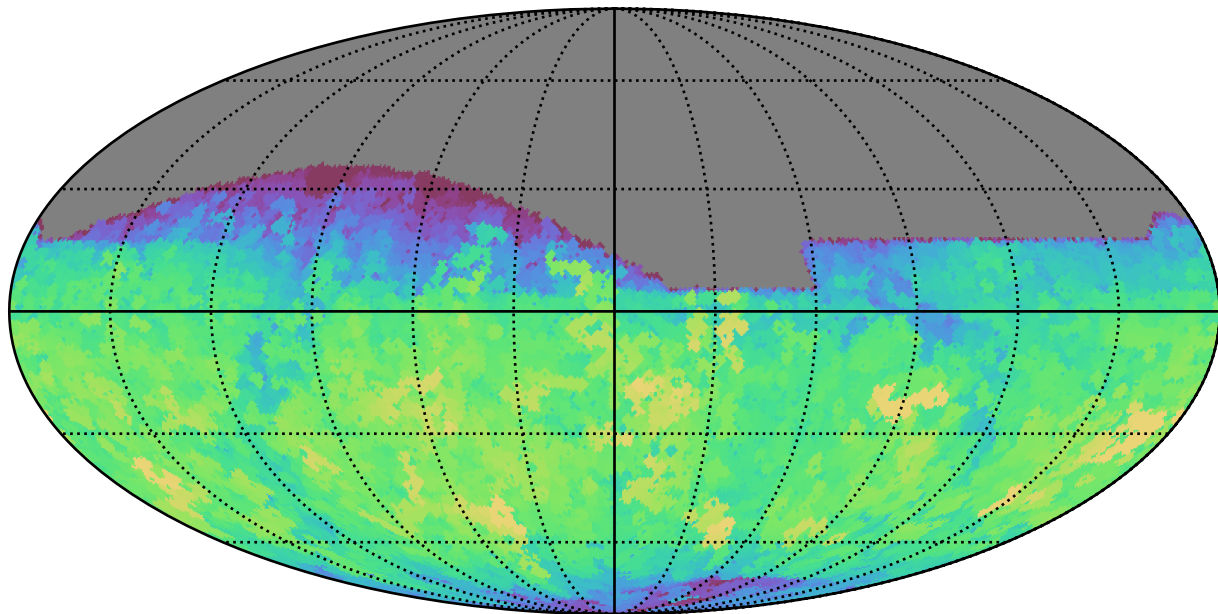
baseline_v3.3_10yrs All sky z band: Max saturation_mag
