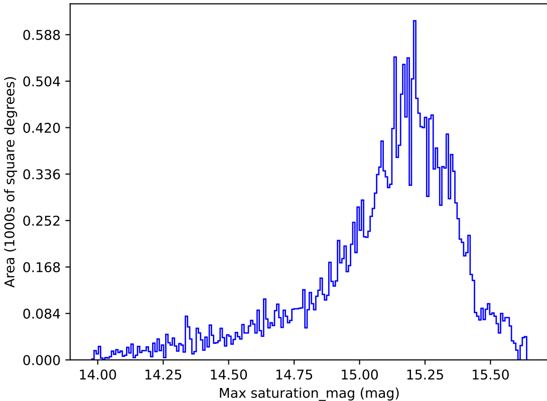
baseline_v3.3_10yrs All sky z band: Max saturation_mag
