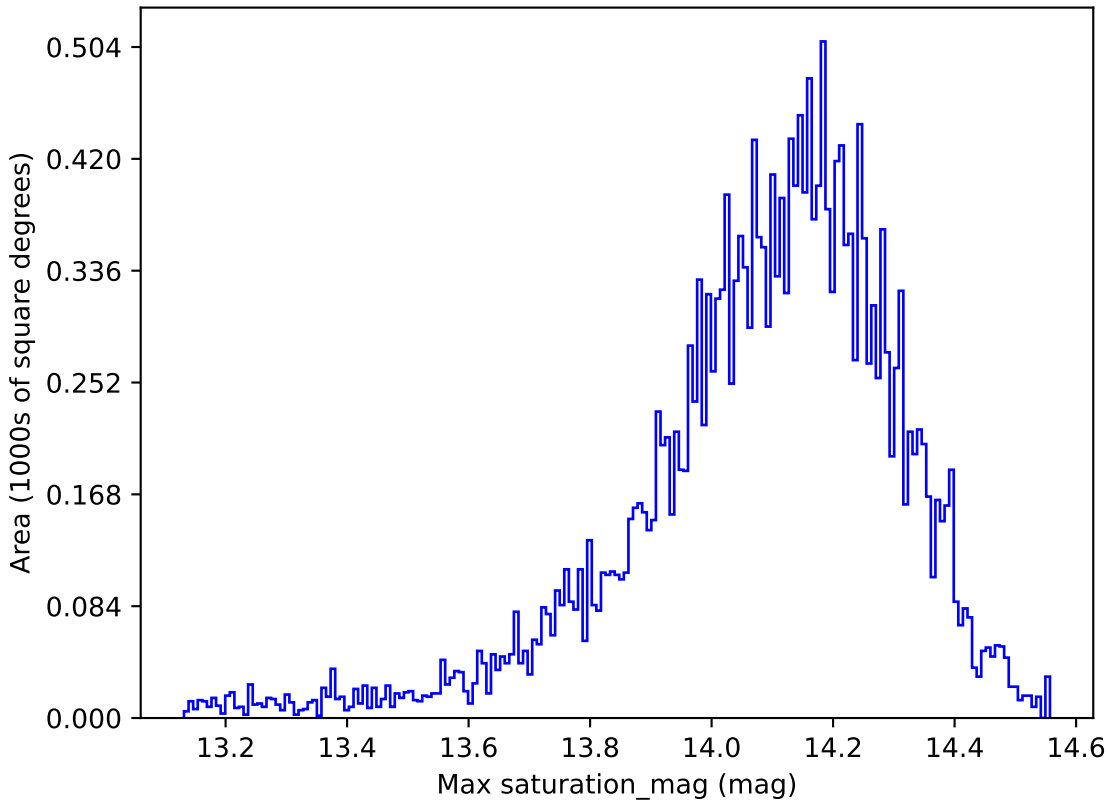
baseline_v3.3_10yrs All sky y band: Max saturation_mag
