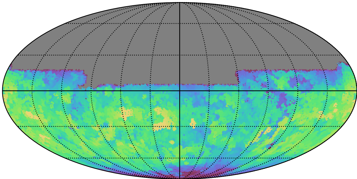
baseline_v3.3_10yrs All sky u band: Max saturation_mag
