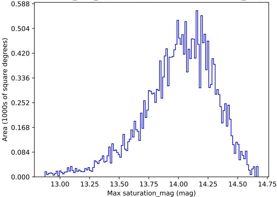
baseline_v3.3_10yrs All sky u band: Max saturation_mag
