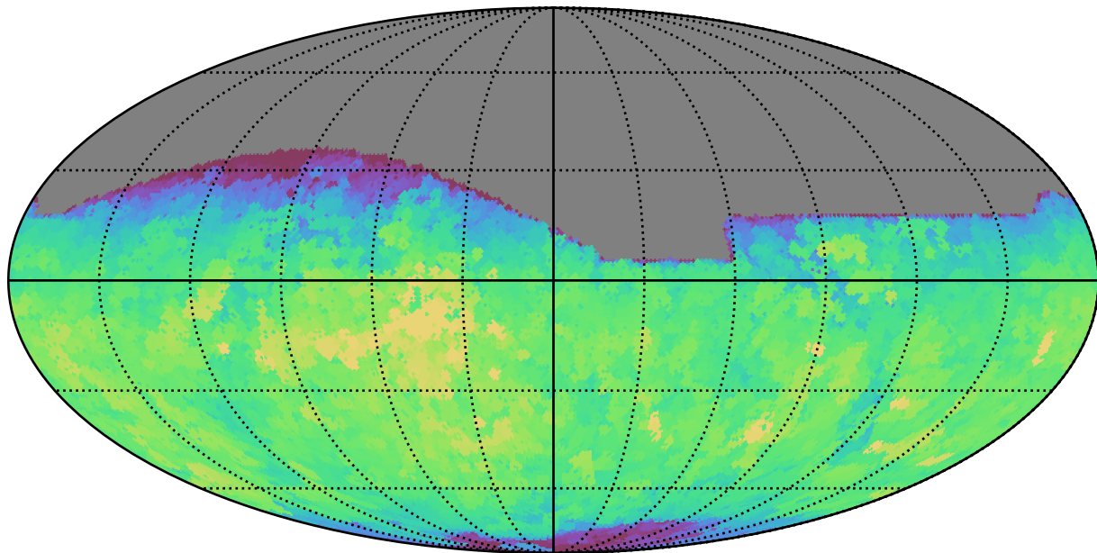
baseline_v3.3_10yrs All sky r band: Max saturation_mag
