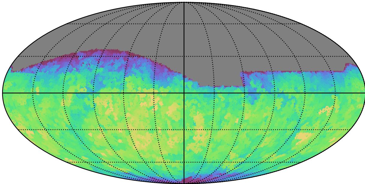
baseline_v3.3_10yrs All sky i band: Max saturation_mag
